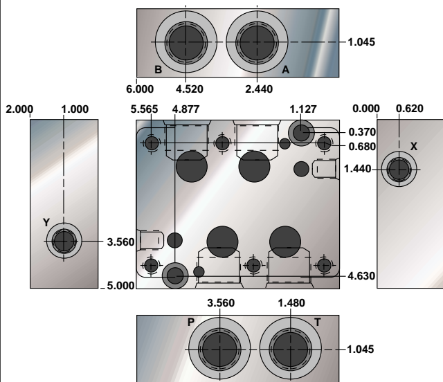
DO8 Subplate
