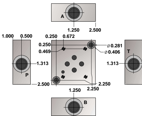
DO3 Subplate
