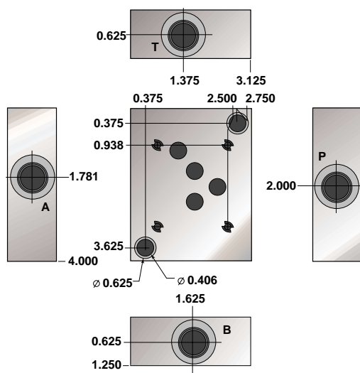
DO5 Subplate
